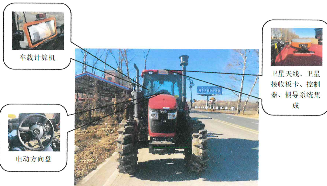
A100BD-2. 5GD 型北斗导航农机自动驾驶系统
